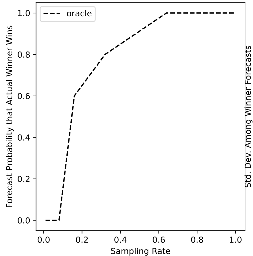
ers-86 Forecast
