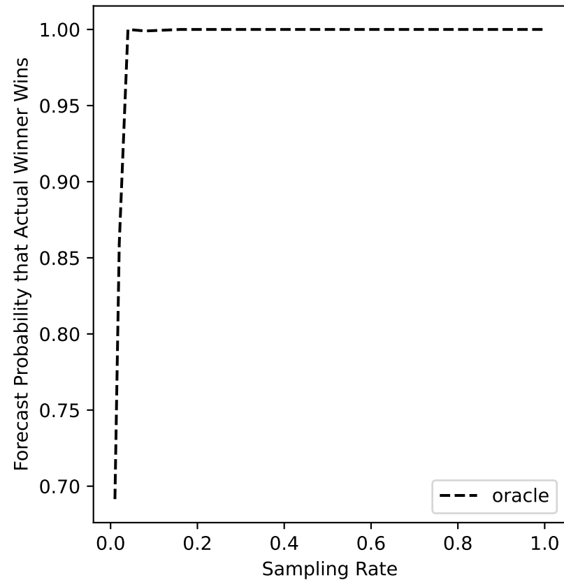
ers-03 Forecast
