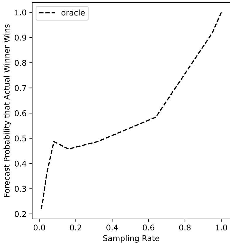
ers-14 Forecast
