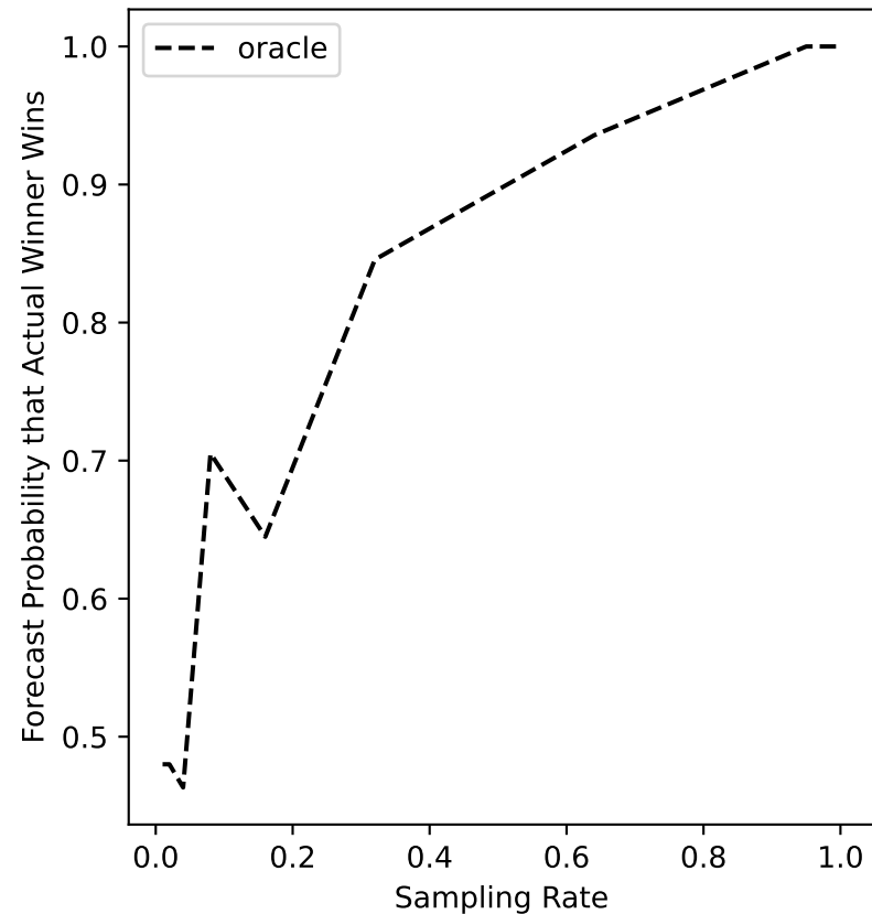
ers-17 Forecast
