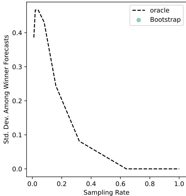
ers-31 Uncertainty
