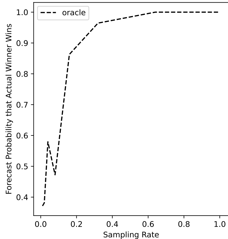
ers-31 Forecast
