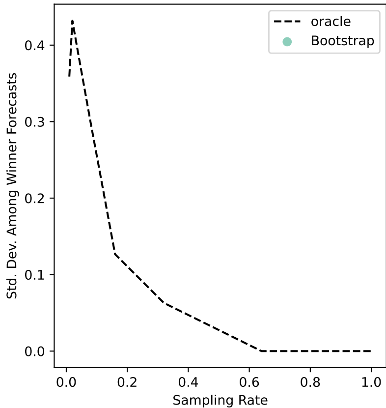
ers-36 Uncertainty
