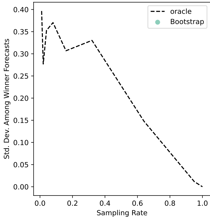
ers-39 Uncertainty
