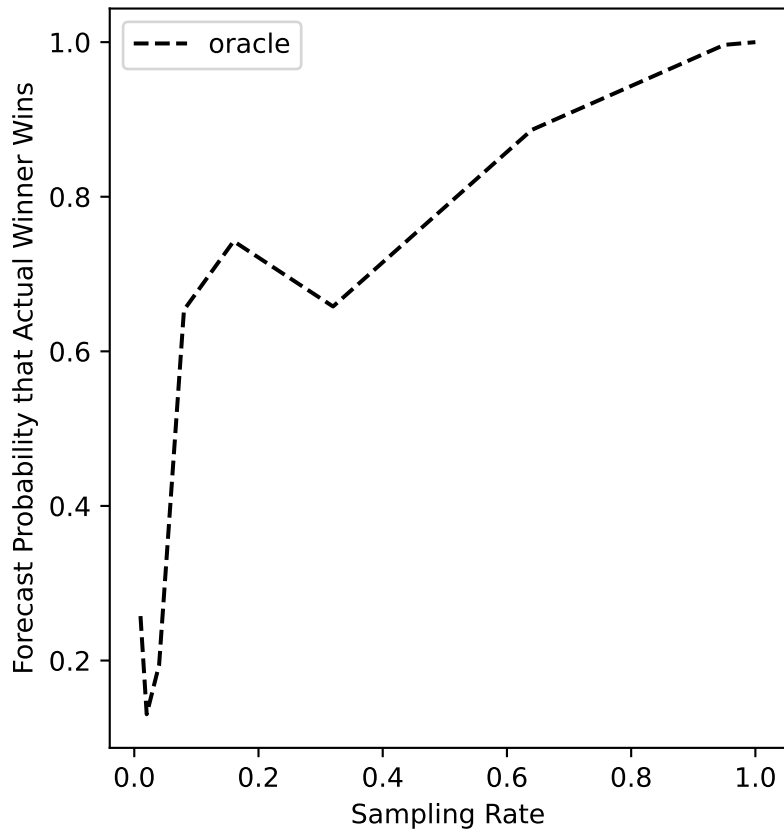
ers-39 Forecast
