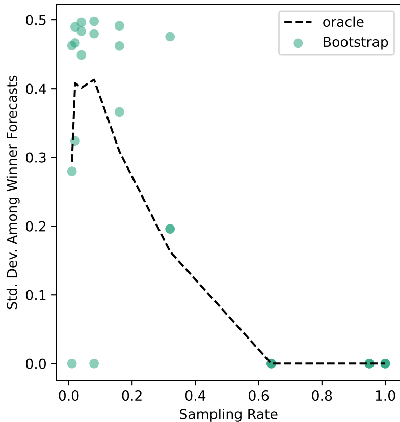
ers-42 Uncertainty
