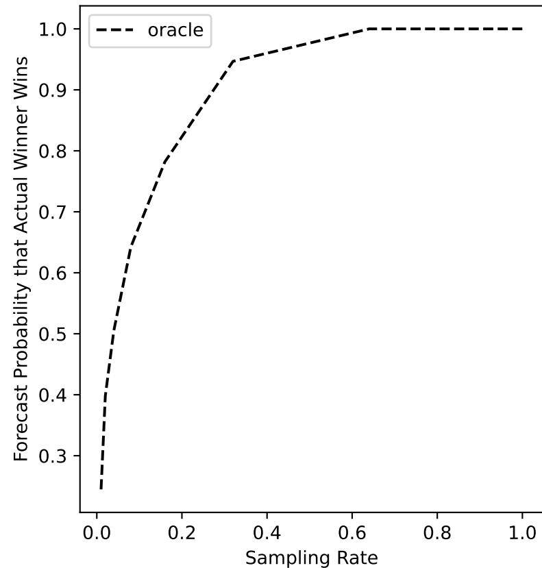
ers-42 Forecast
