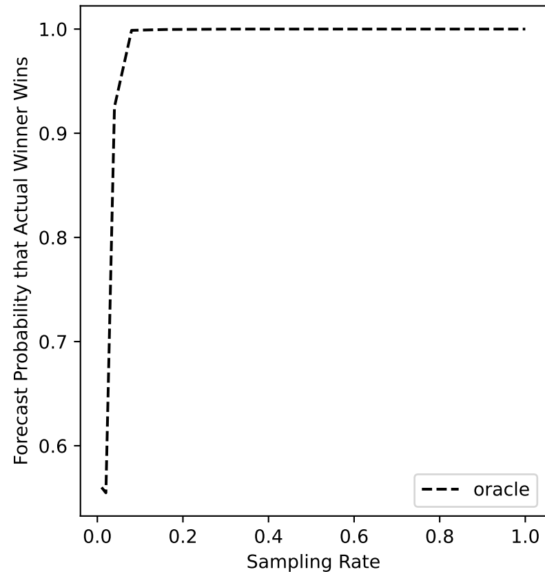
ers-50 Forecast
