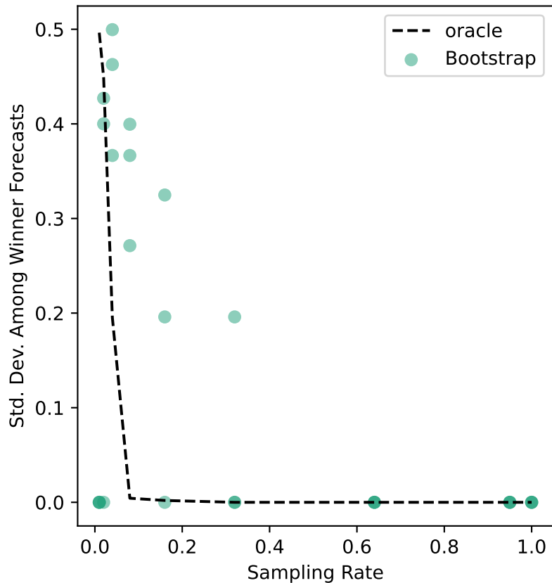
ers-50 Uncertainty
