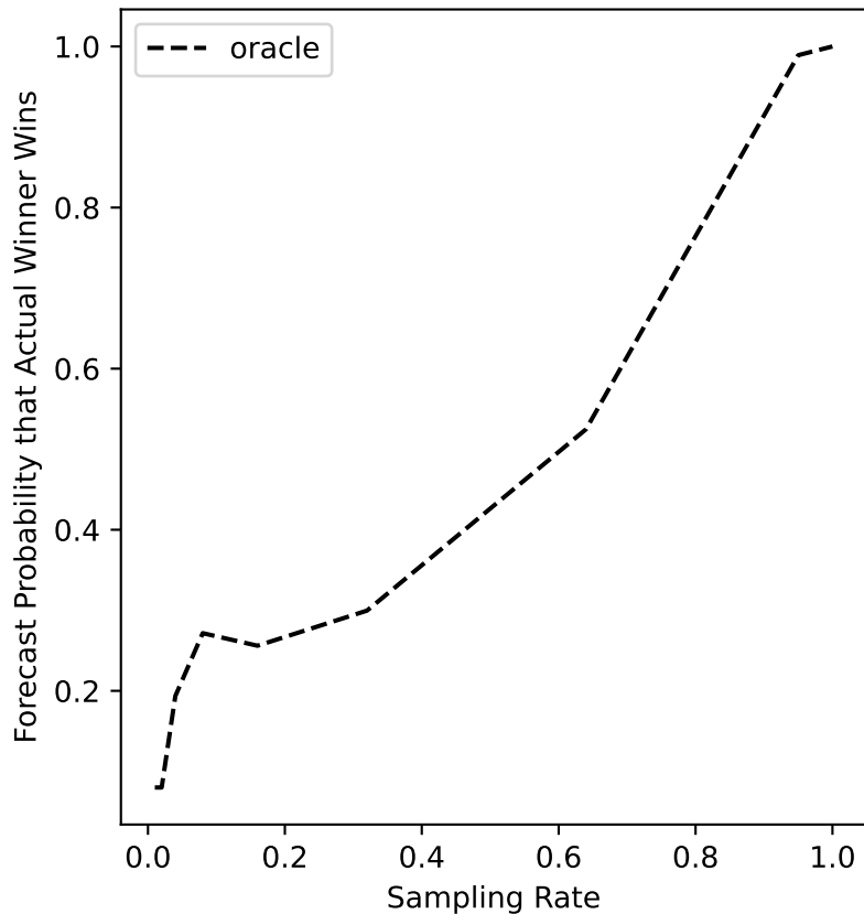
ers-54 Forecast
