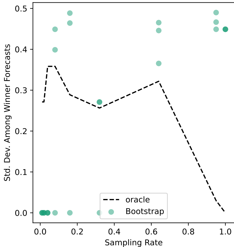
ers-54 Uncertainty
