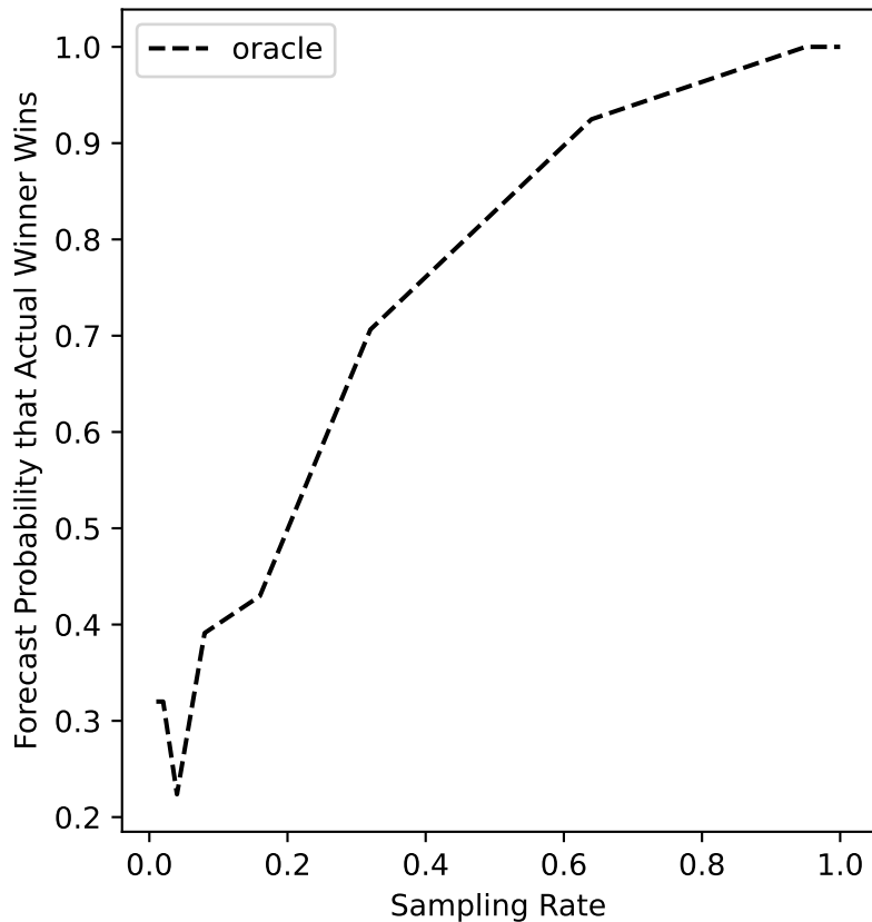
ers-55 Forecast
