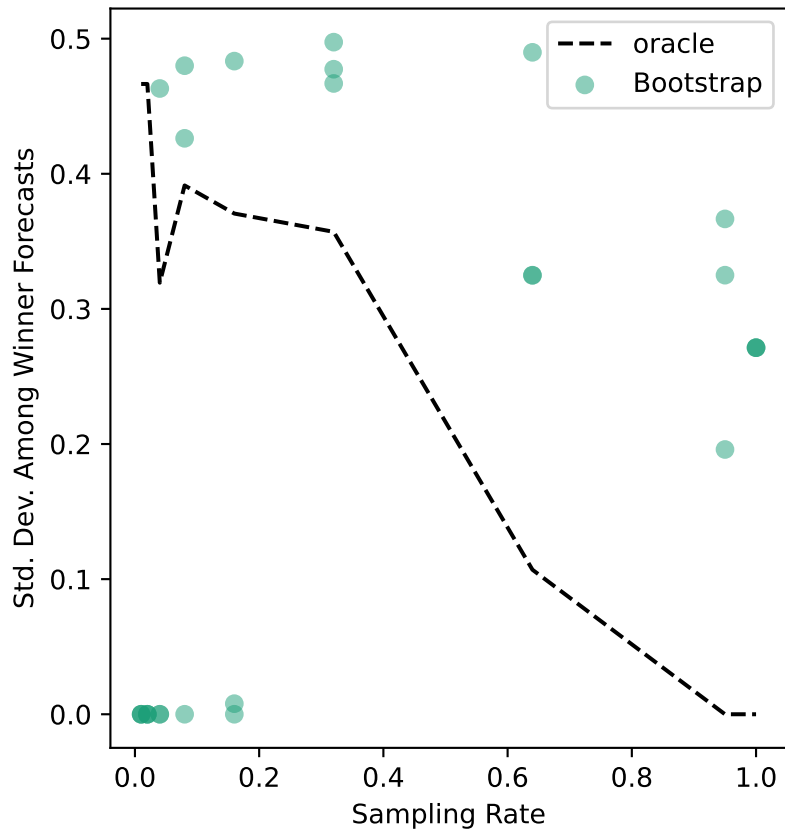
ers-55 Uncertainty
