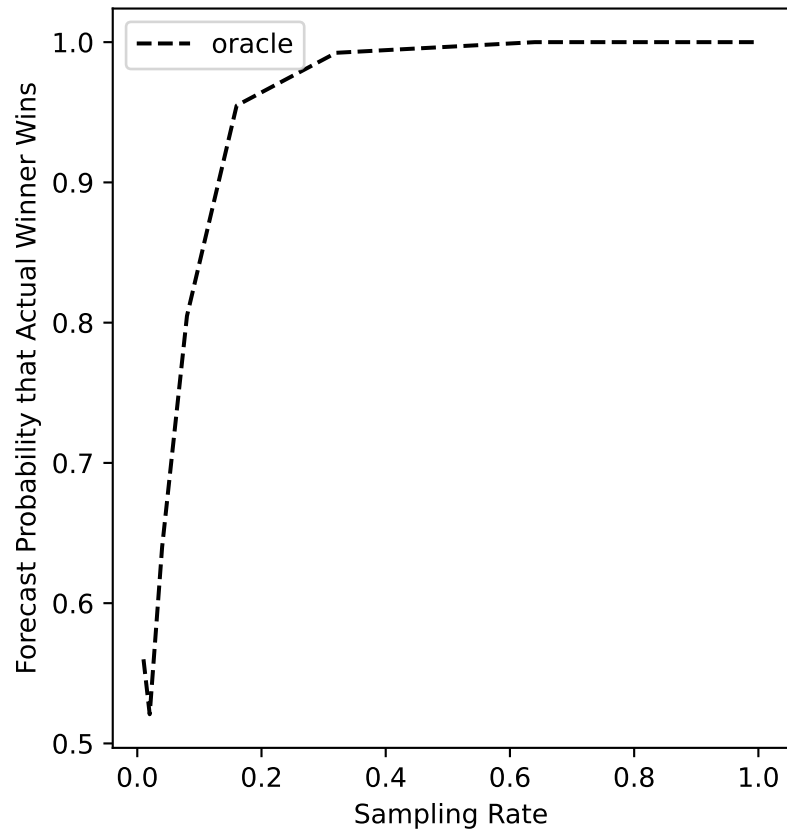
ers-60 Forecast
