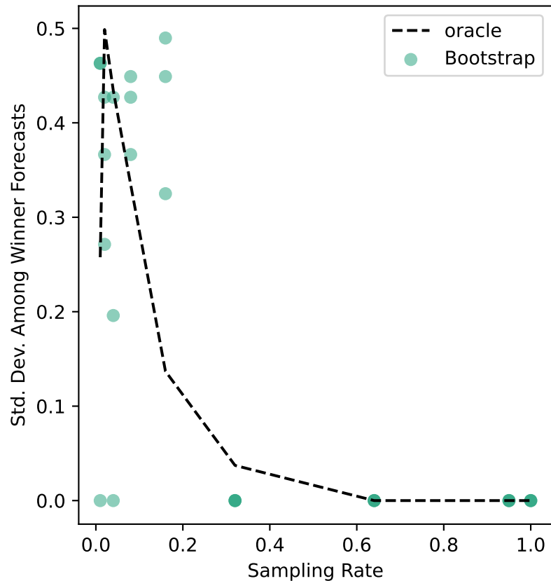
ers-60 Uncertainty
