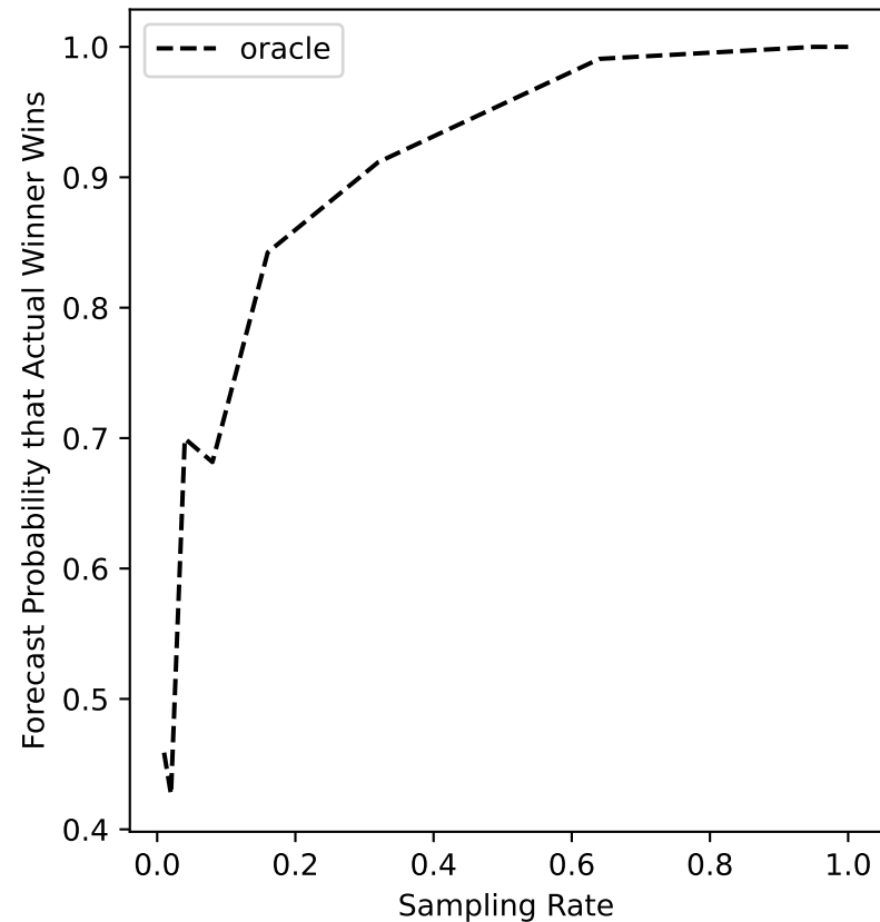
ers-61 Forecast
