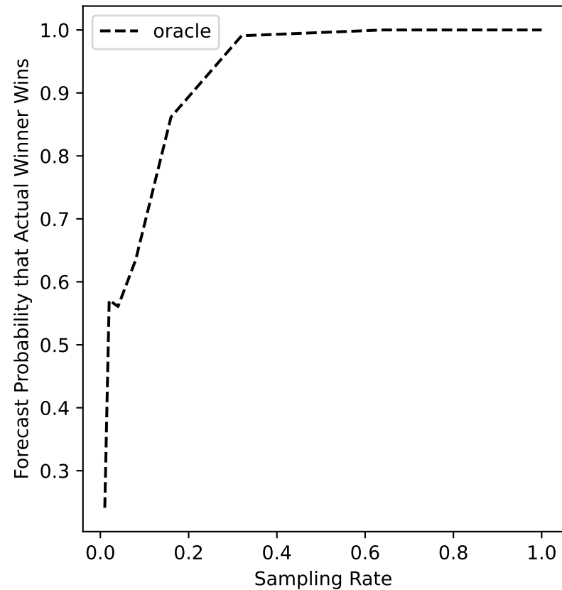
ers-71 Forecast
