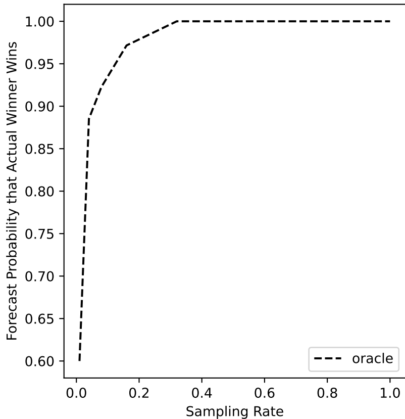
ers-75 Forecast
