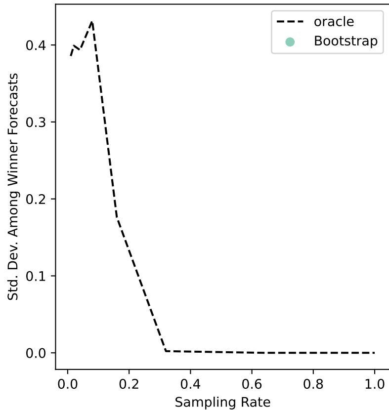
ers-80 Uncertainty
