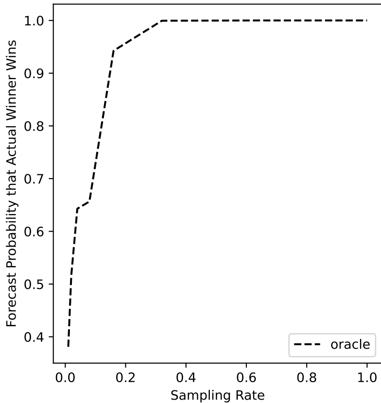
ers-80 Forecast
