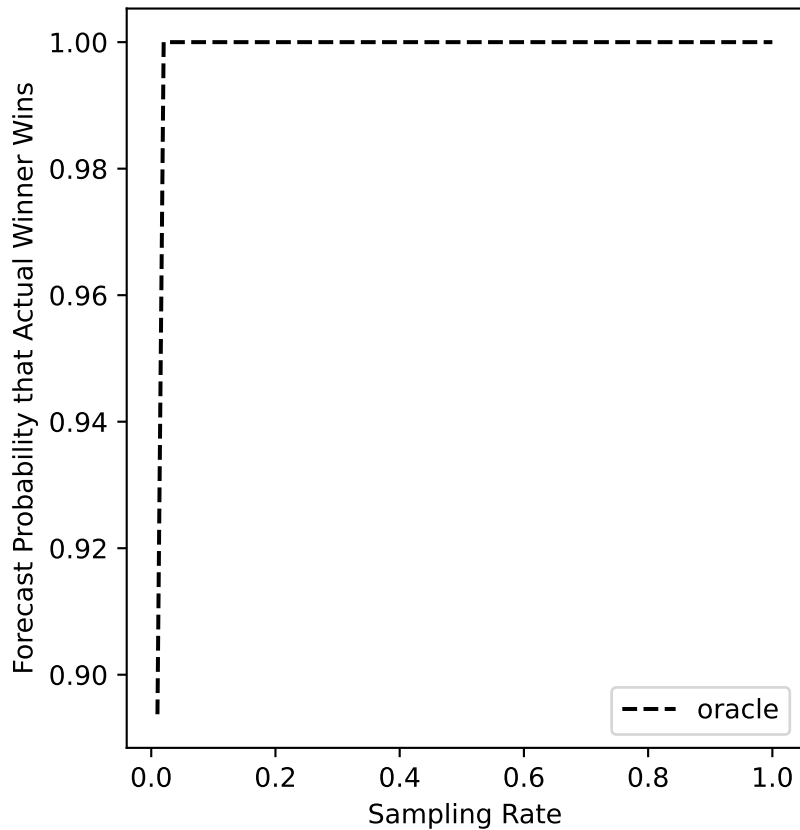
ers-03 Forecast
