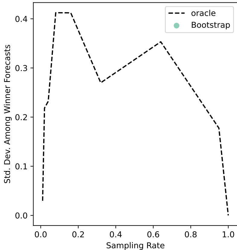
ers-11 Uncertainty
