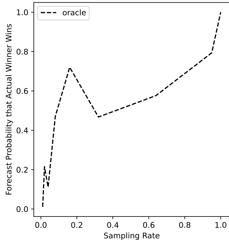
ers-11 Forecast
