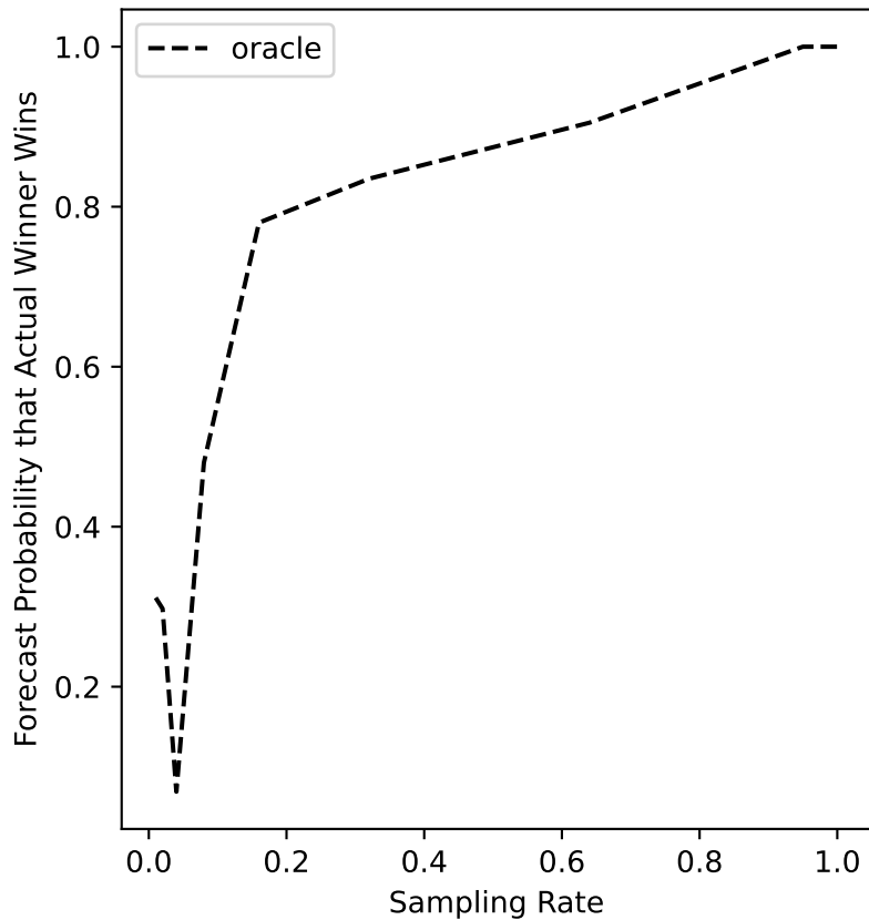
ers-12 Forecast
