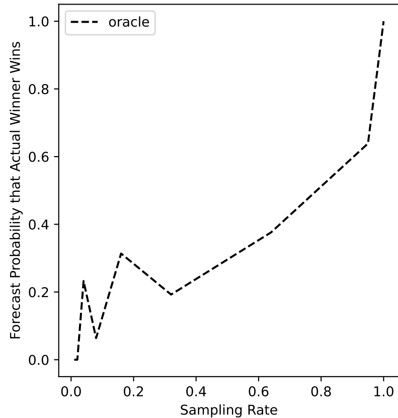
ers-16 Forecast
