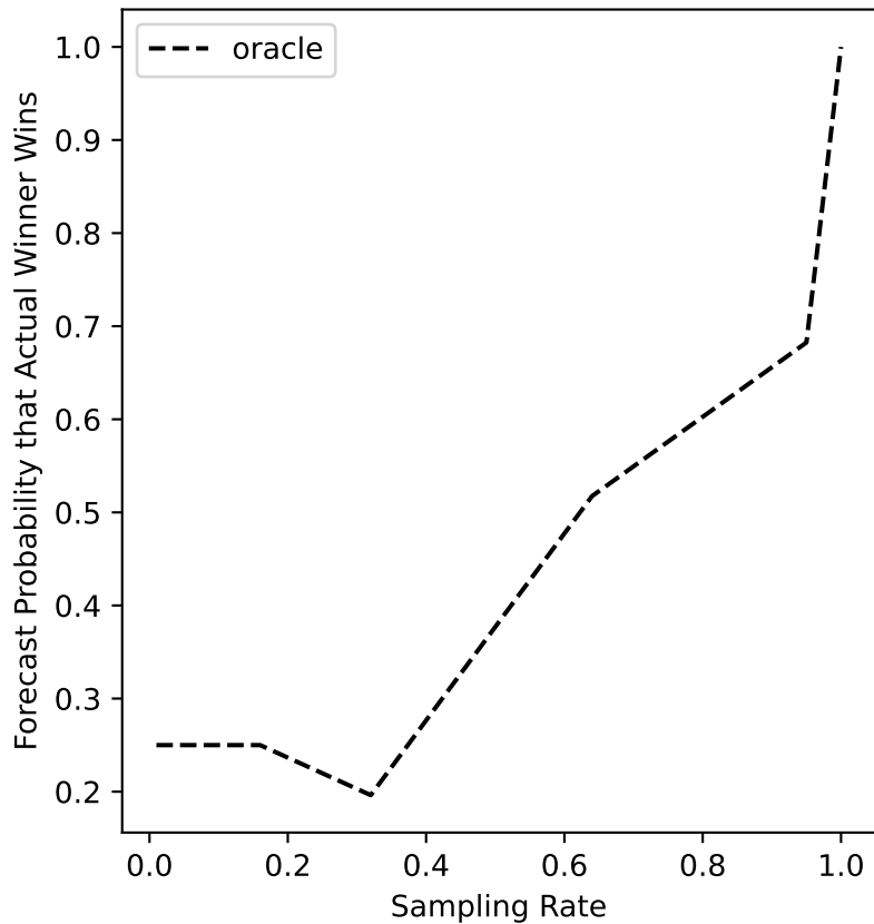
ers-27 Forecast
