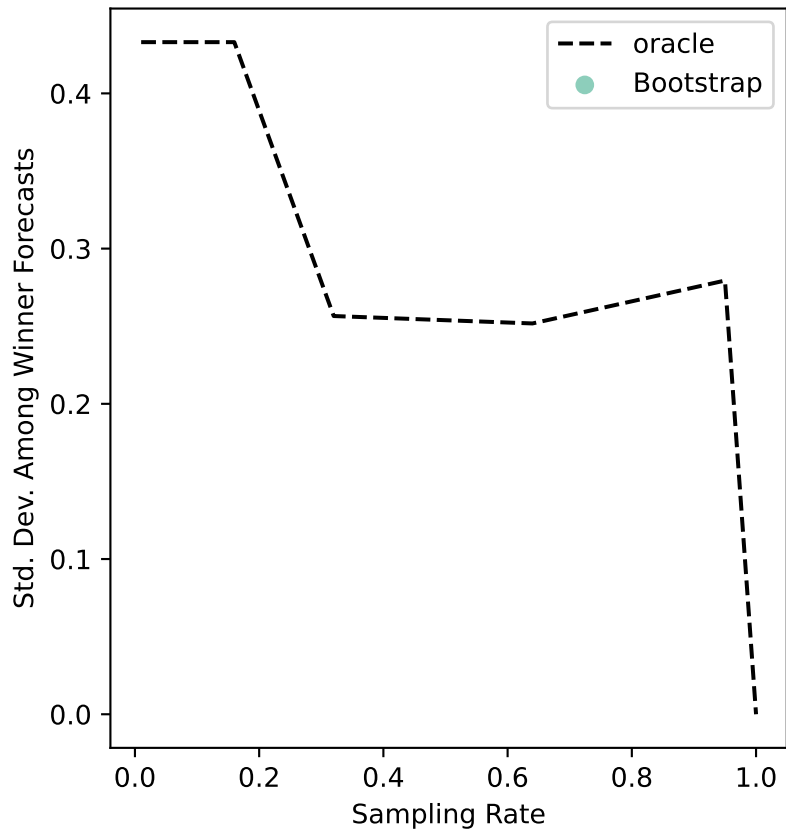
ers-27 Uncertainty
