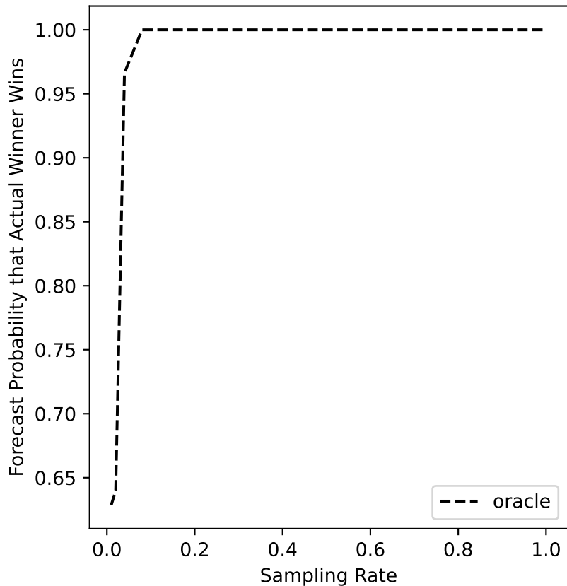
ers-33 Forecast
