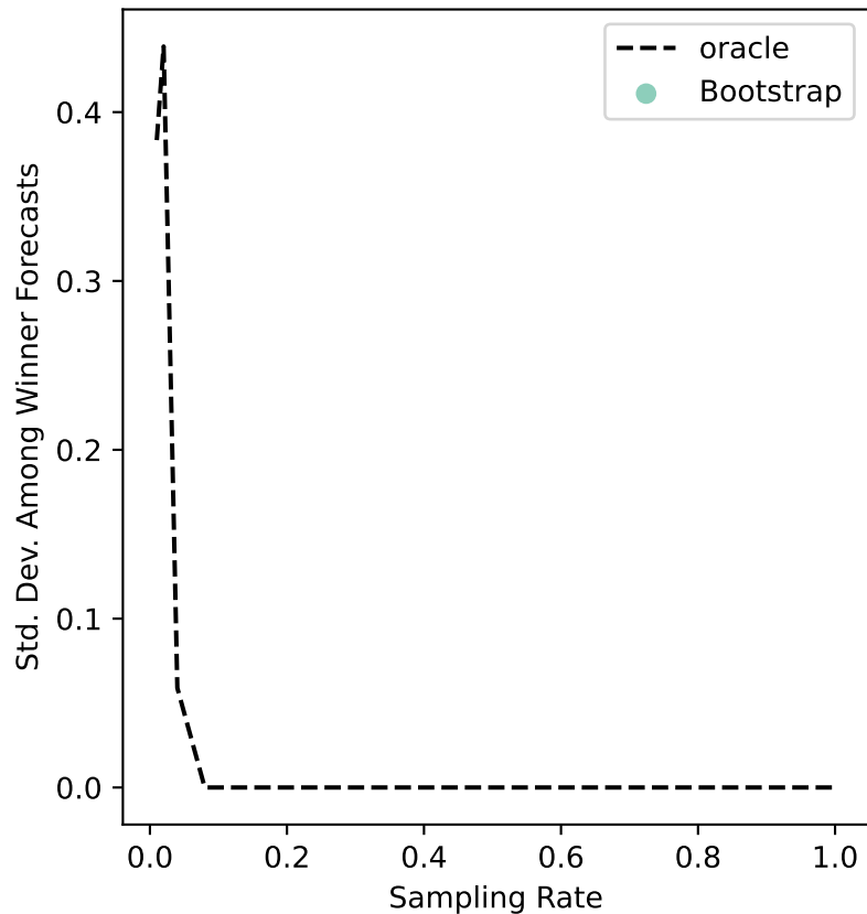
ers-33 Uncertainty
