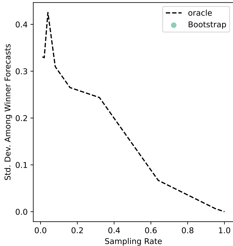
ers-39 Uncertainty
