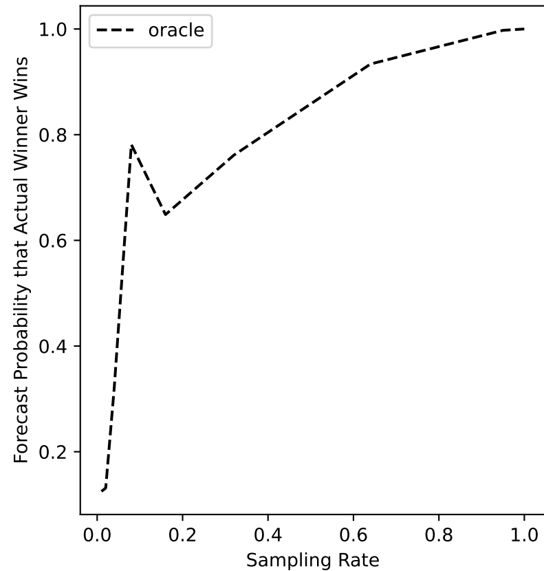
ers-39 Forecast
