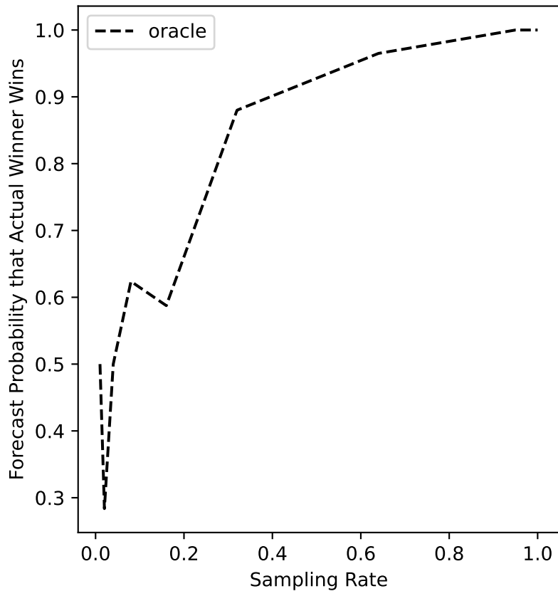
ers-45 Forecast
