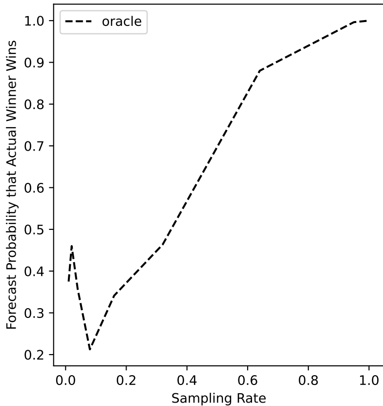
ers-47 Forecast
