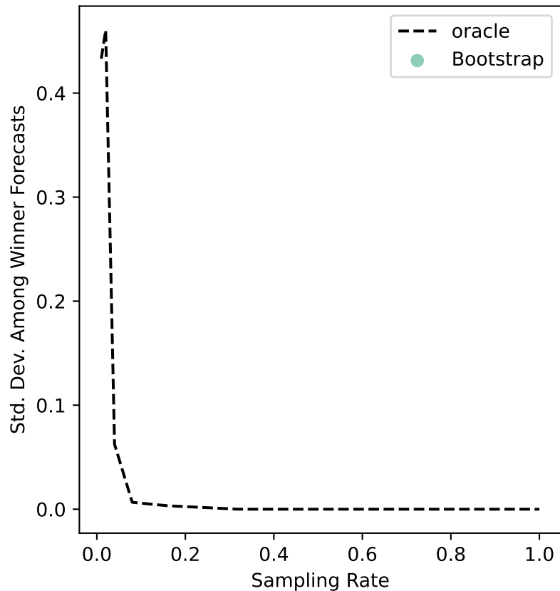
ers-50 Uncertainty
