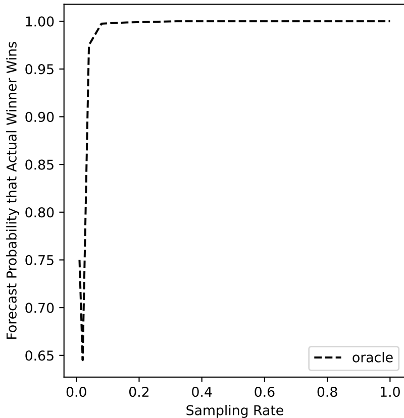
ers-50 Forecast
