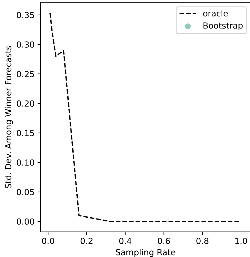
ers-56 Uncertainty
