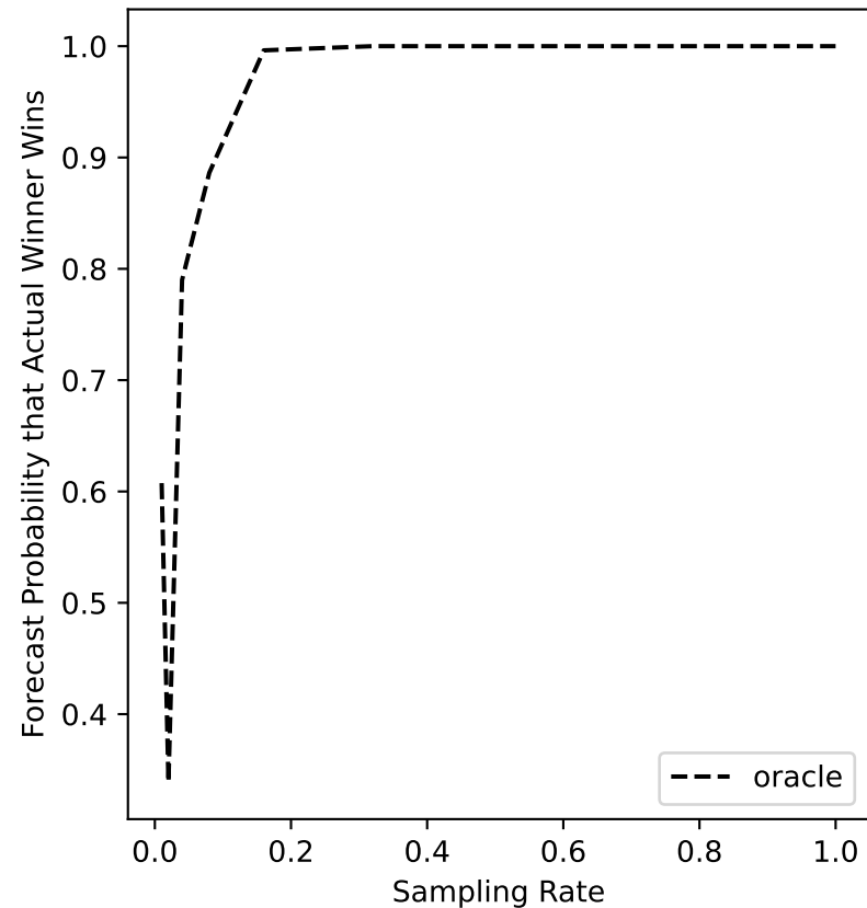
ers-56 Forecast
