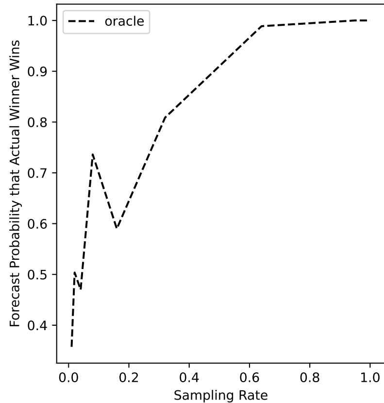
ers-62 Forecast
