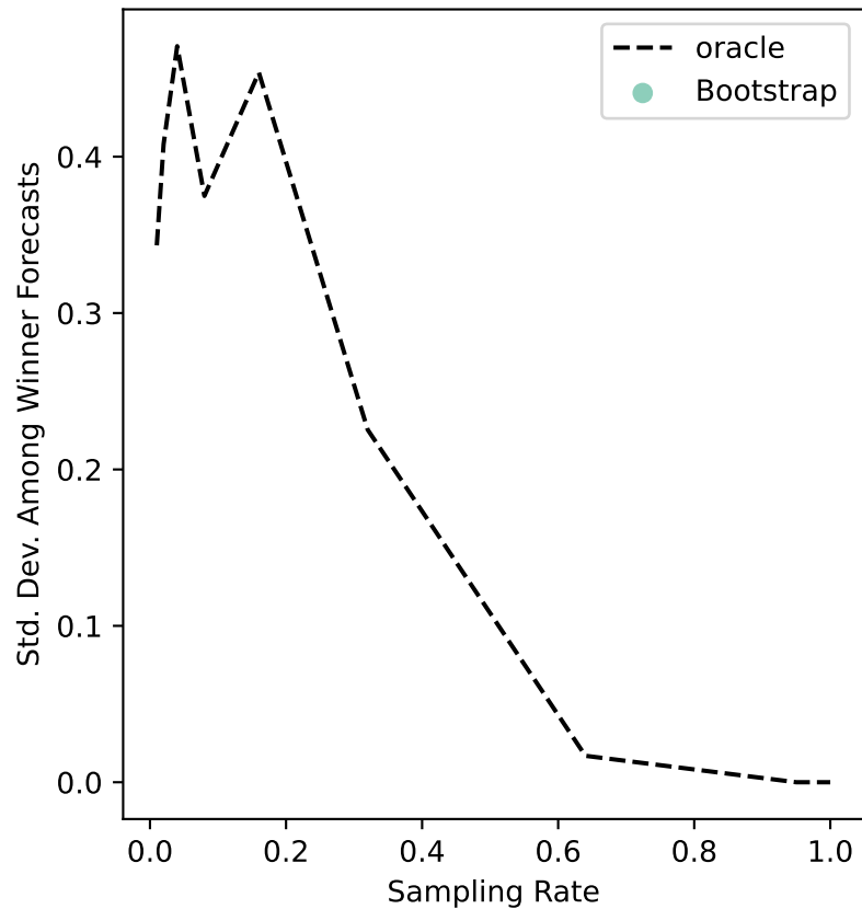
ers-62 Uncertainty
