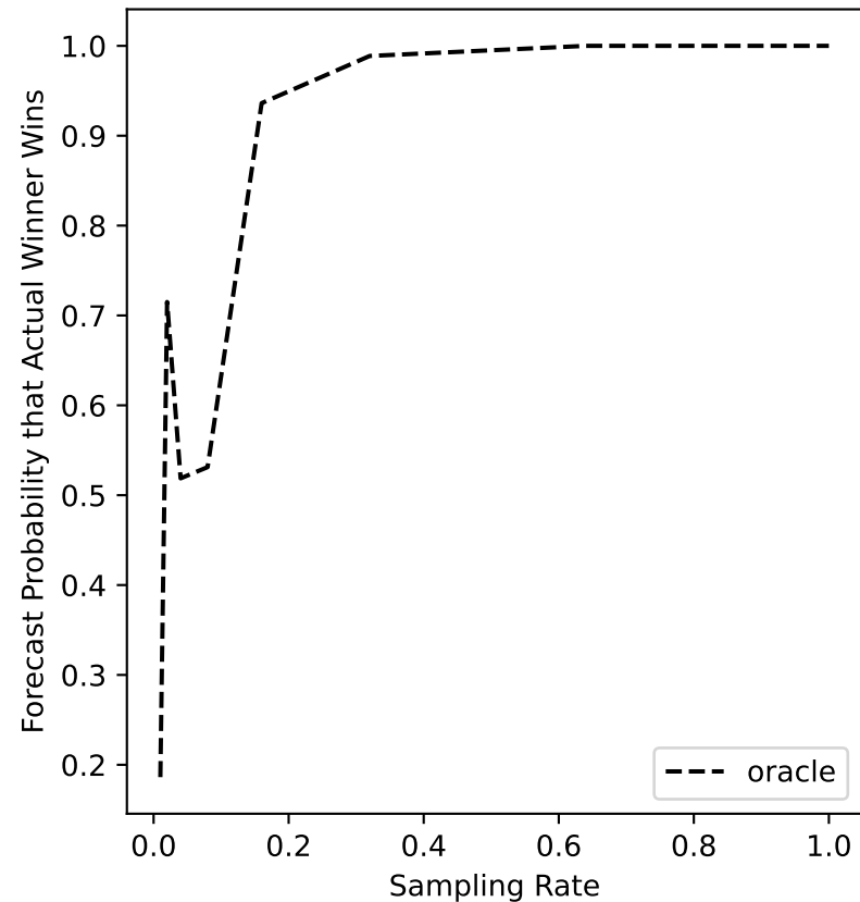
ers-71 Forecast
