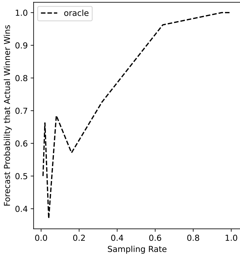
ers-72 Forecast
