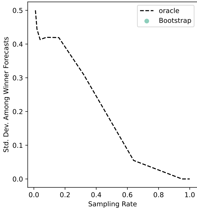
ers-72 Uncertainty
