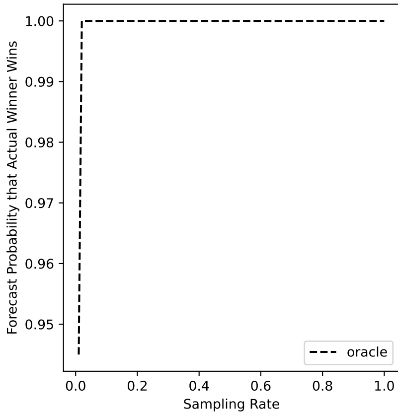
ers-77 Forecast
