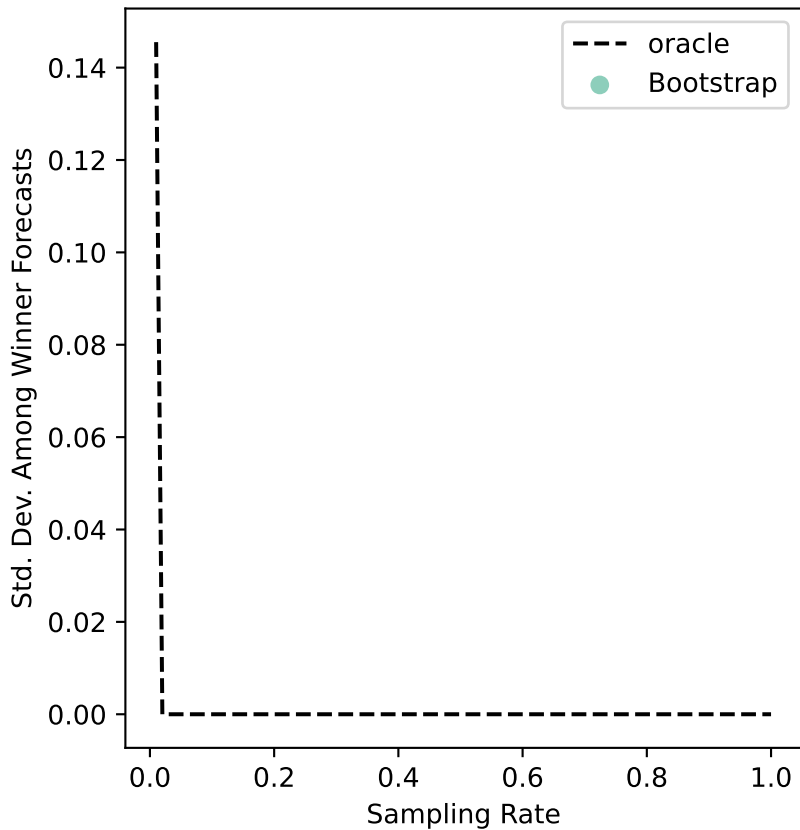
ers-77 Uncertainty
