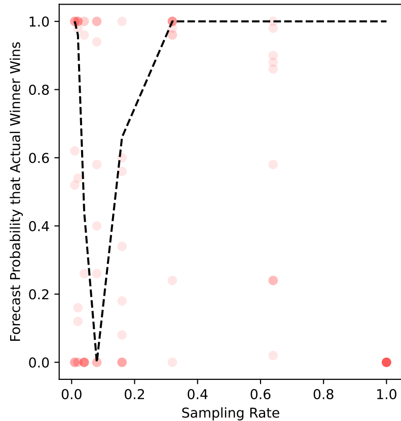
ers-13 Forecast
