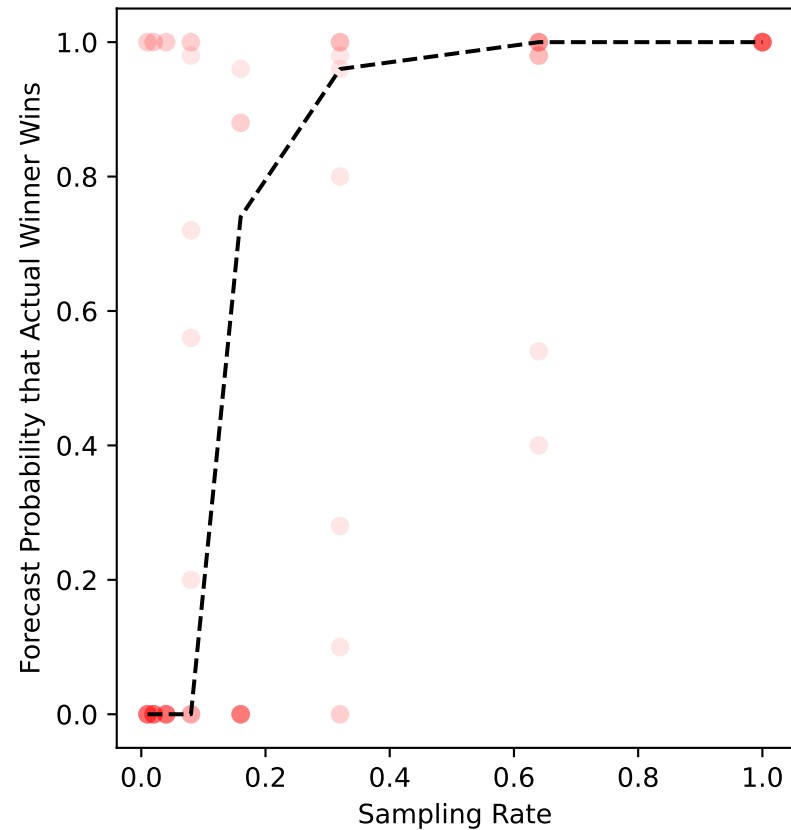
ers-15 Forecast
