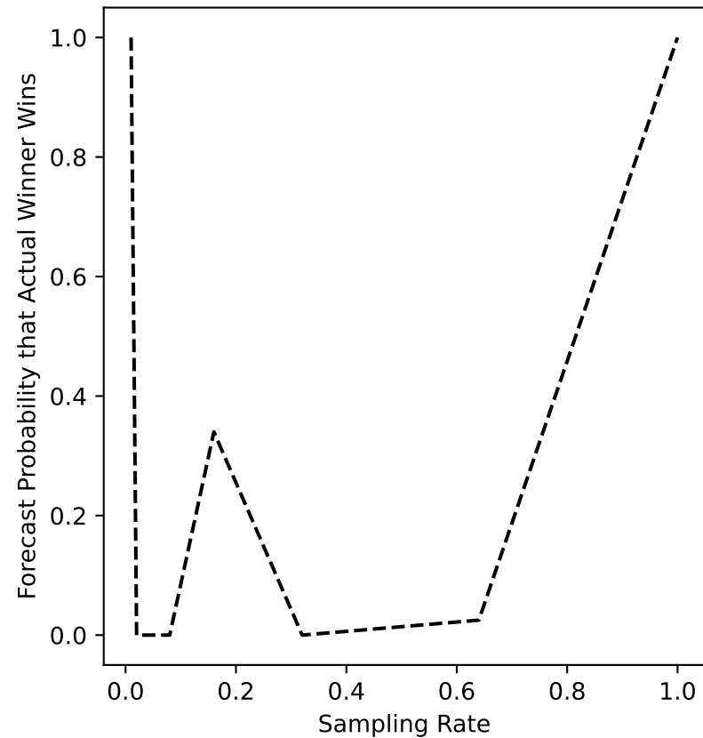
ers-19 Forecast
