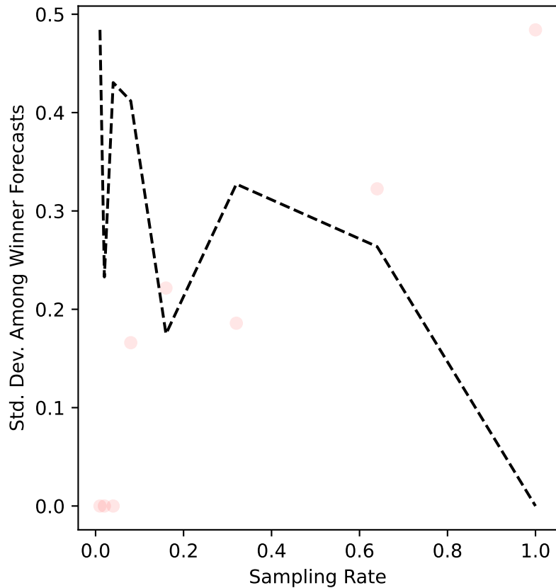
ers-19 Uncertainty
