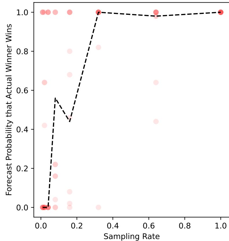
ers-26 Forecast
