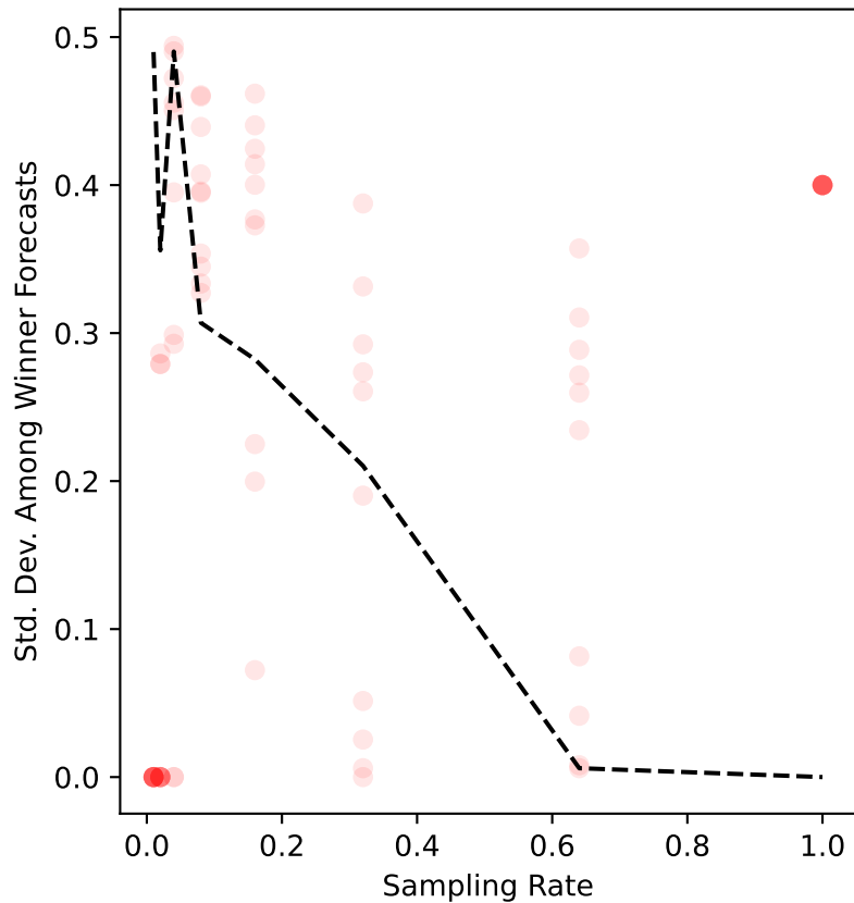
ers-26 Uncertainty
