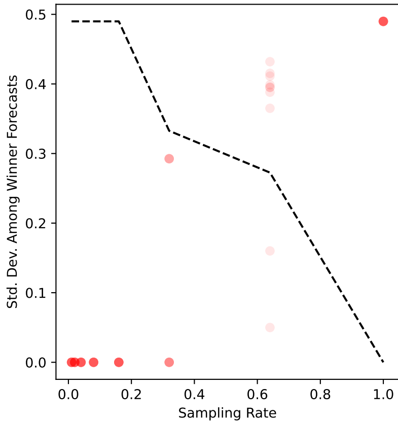
ers-27 Uncertainty
