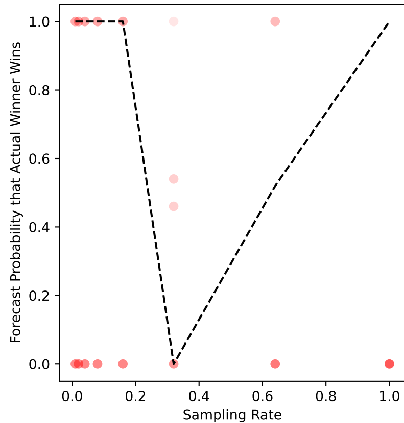
ers-27 Forecast
