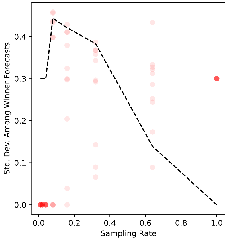
ers-35 Uncertainty
