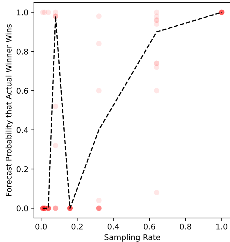
ers-35 Forecast
