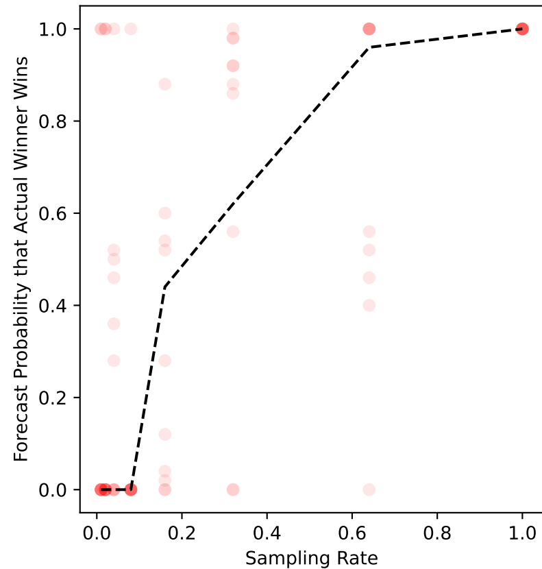
ers-55 Forecast
