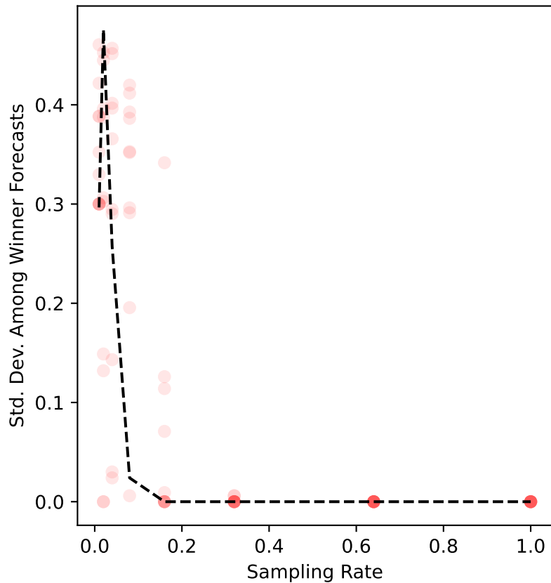
ers-56 Uncertainty
