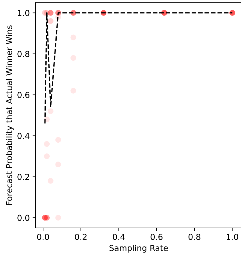
ers-56 Forecast
