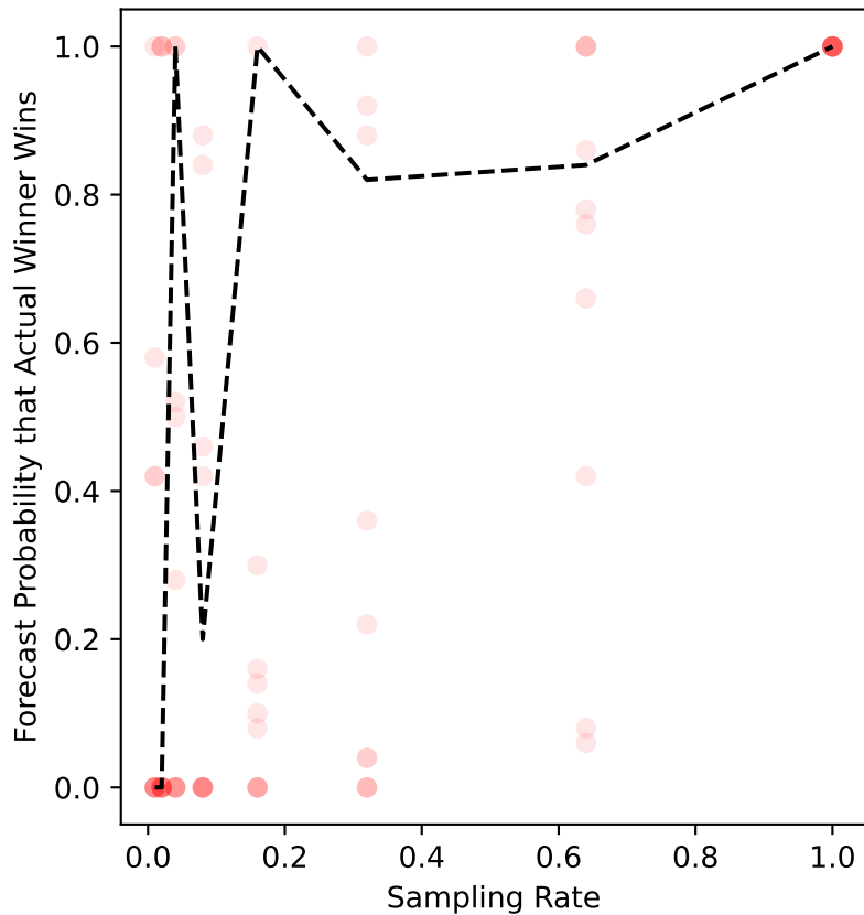
ers-85 Forecast
