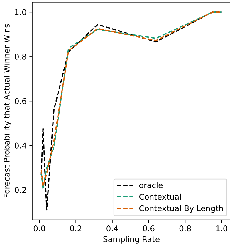
ers-12 Forecast
