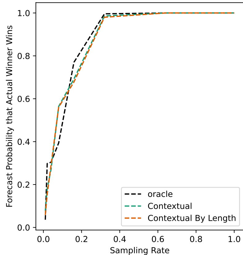
ers-65 Forecast
