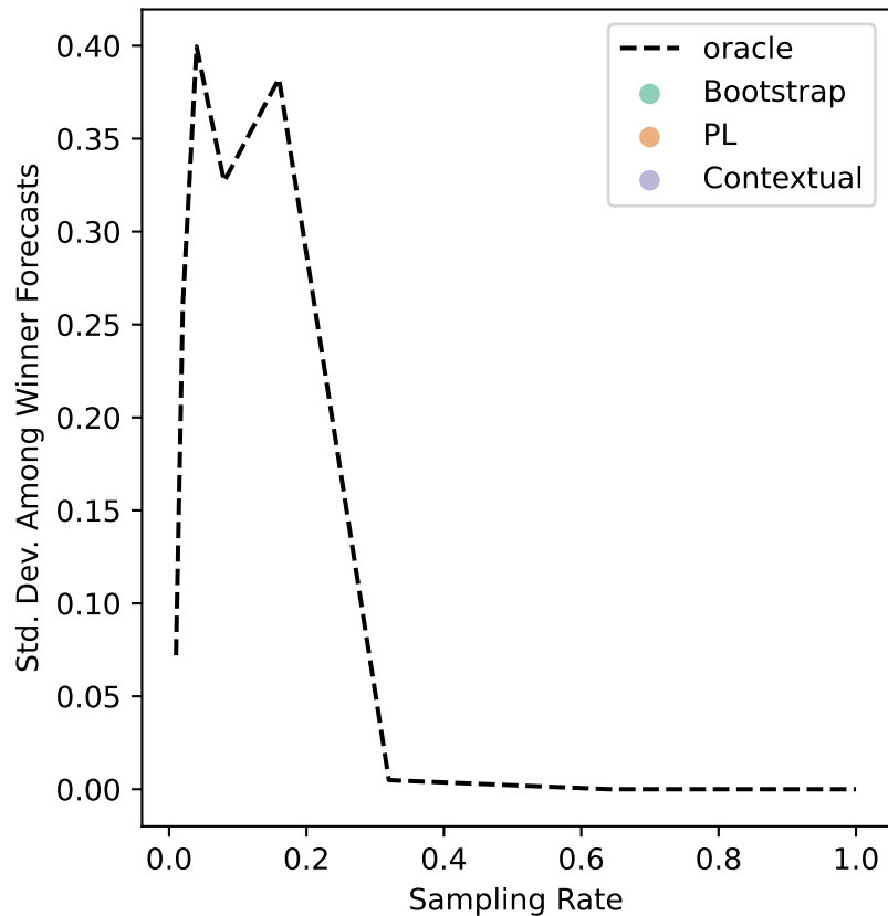
ers-65 Uncertainty
