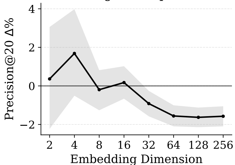
MovieLens-1M Target Group: 56
