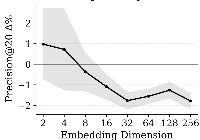
MovieLens-1M Target Group: 45
