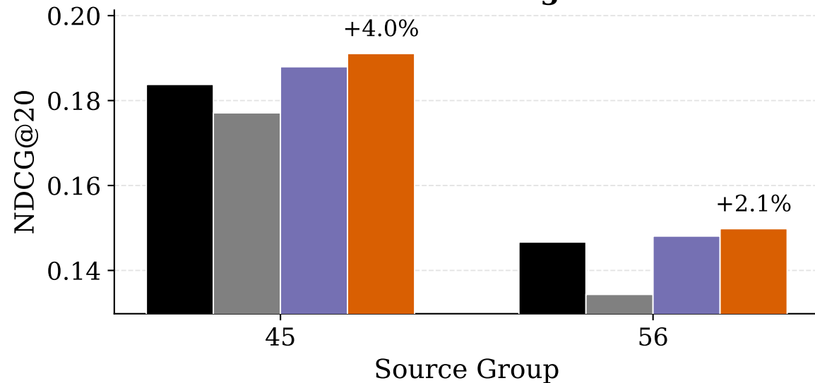
MovieLens-1M LightGCN
