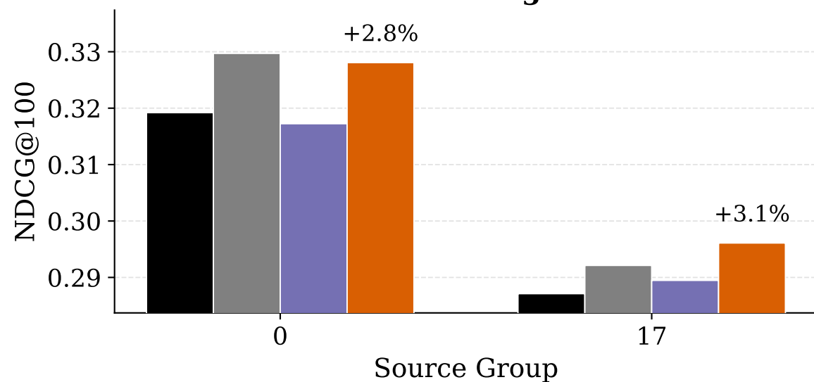
LastFM-Asia LightGCN
