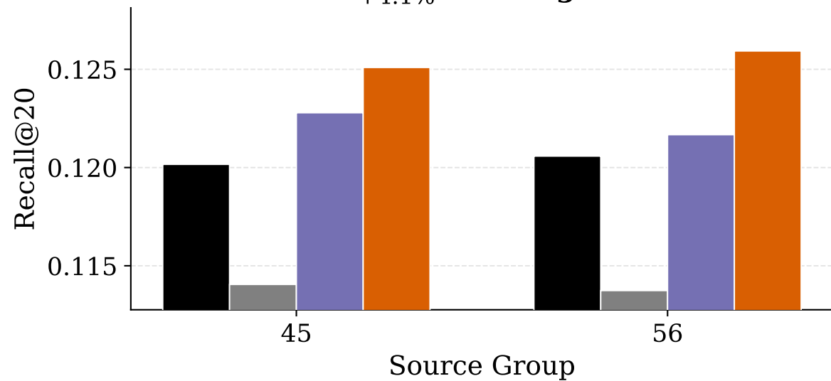
MovieLens-1M LightGCN
