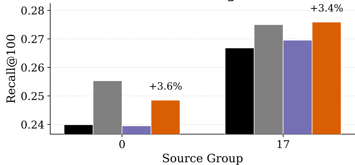
LastFM-Asia LightGCN
