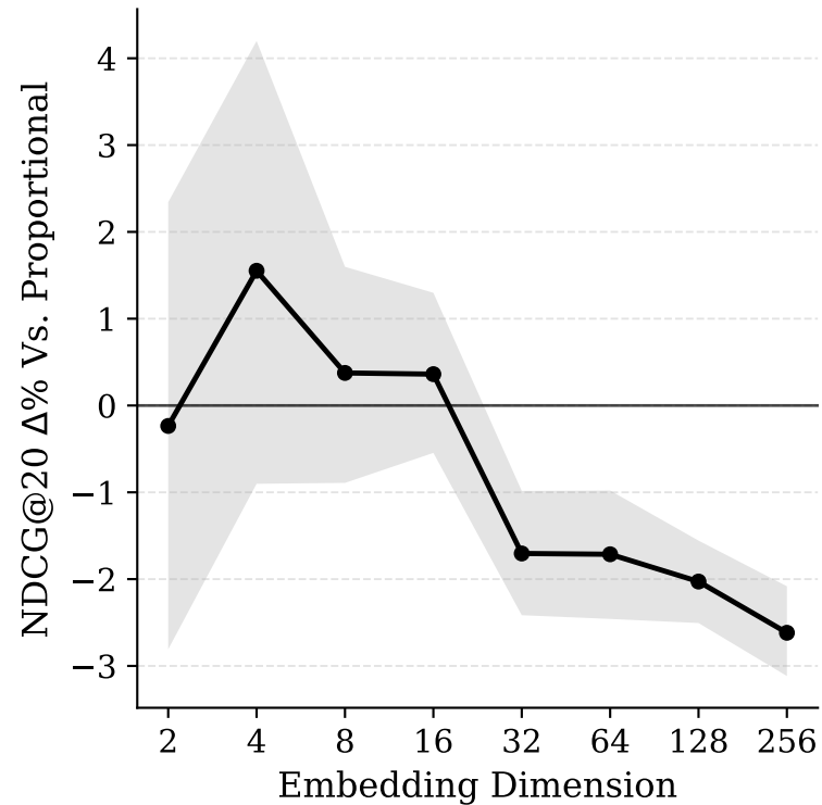
MovieLens-1M Source Group: 56
