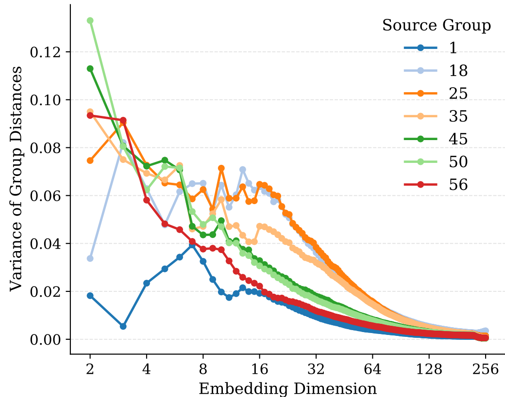
MovieLens-1M
