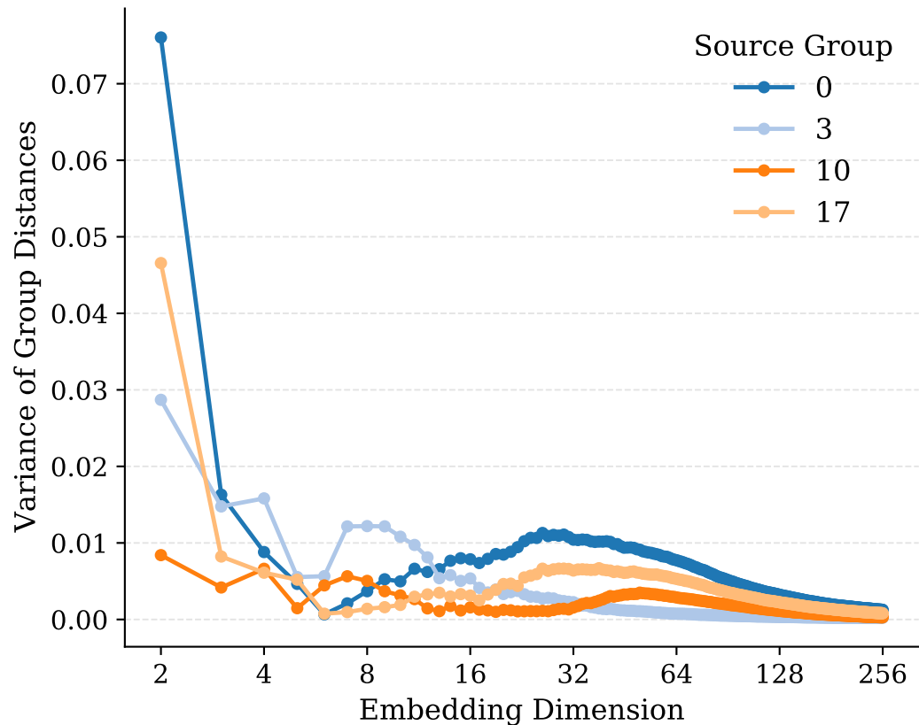
LastFM-Asia
