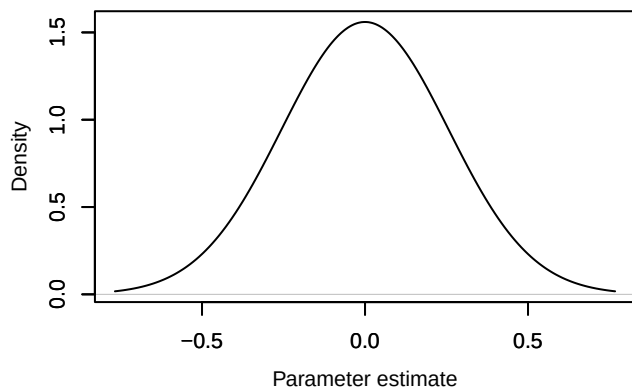
Density – beta.ranef.categ.in_AP[18,1]
