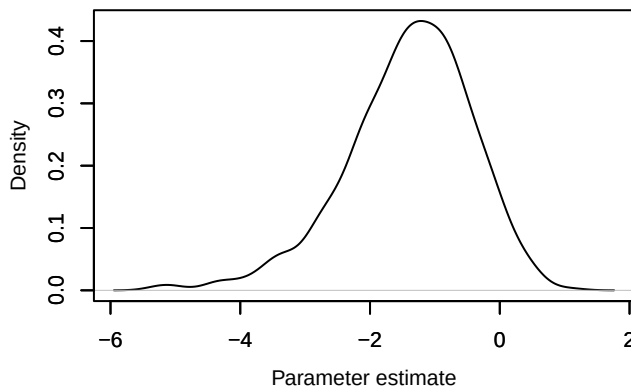
Density – beta.ranef.category.in_AP[10,2]
