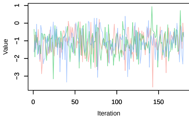
Trace – alpha0[9]
