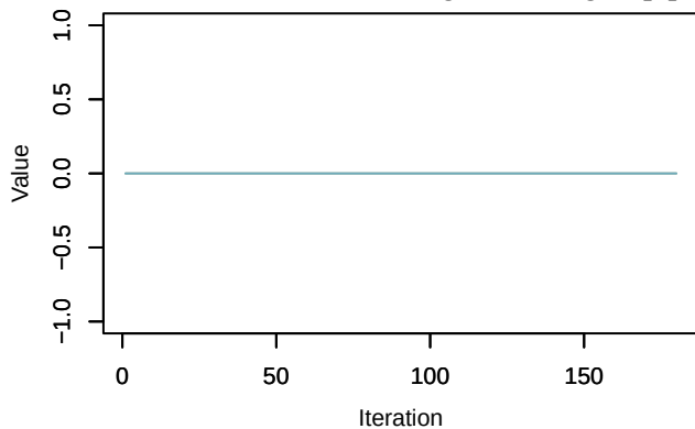
Trace – beta.ranef.categ.in_AP.sigma[2]
