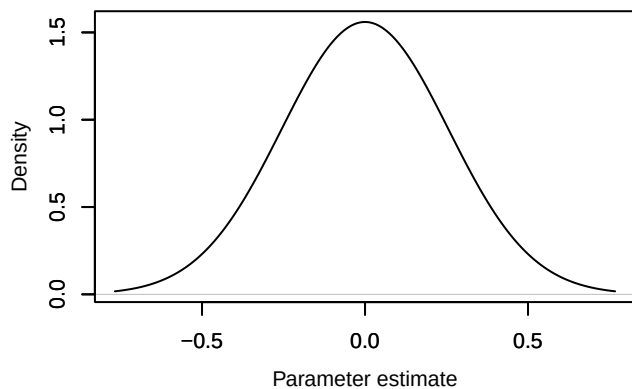
Density – beta.ranef.categ.in_AP[18,1]
