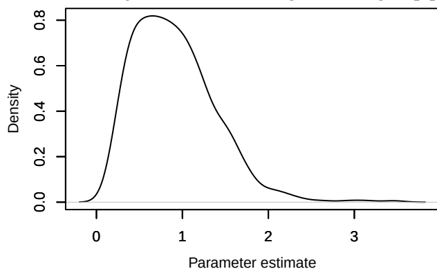
Density – beta.ranef.categ.in_AP.sigma[2]
