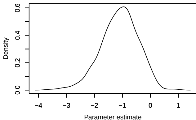
Density – alpha0[9]
