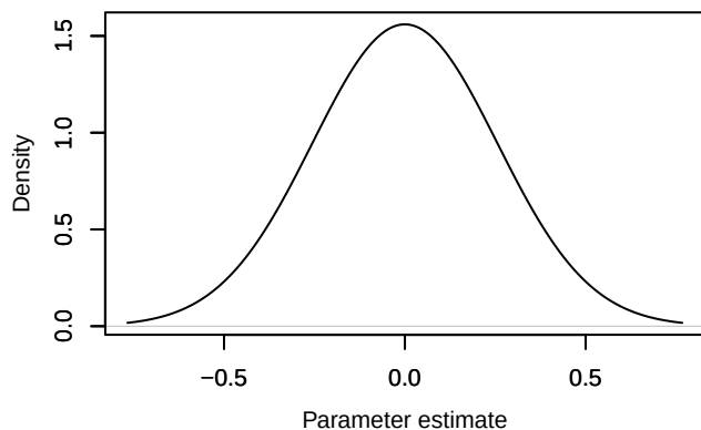
Density – beta.ranef.category.in_AP.mean[1]
