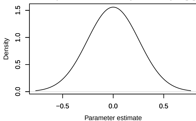
Density – beta.ranef.categ.in_AP.sigma[2]
