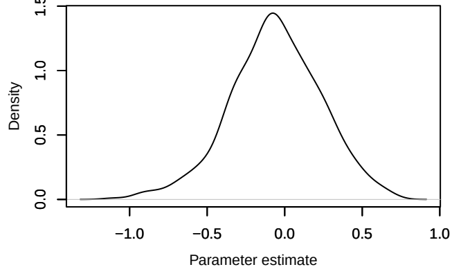
Density – beta.ranef.cont.elev[23]
