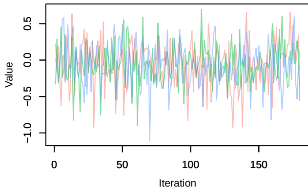
Trace – beta.ranef.cont.elev[23]
