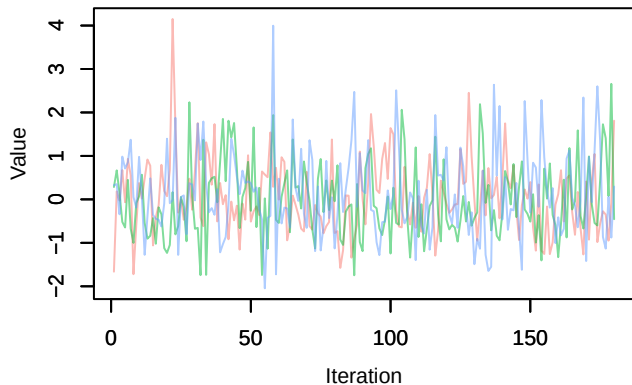
Trace – beta0[23]
