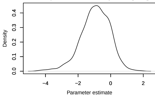
Density – beta.ranef.category.in_AP.mean[1]
