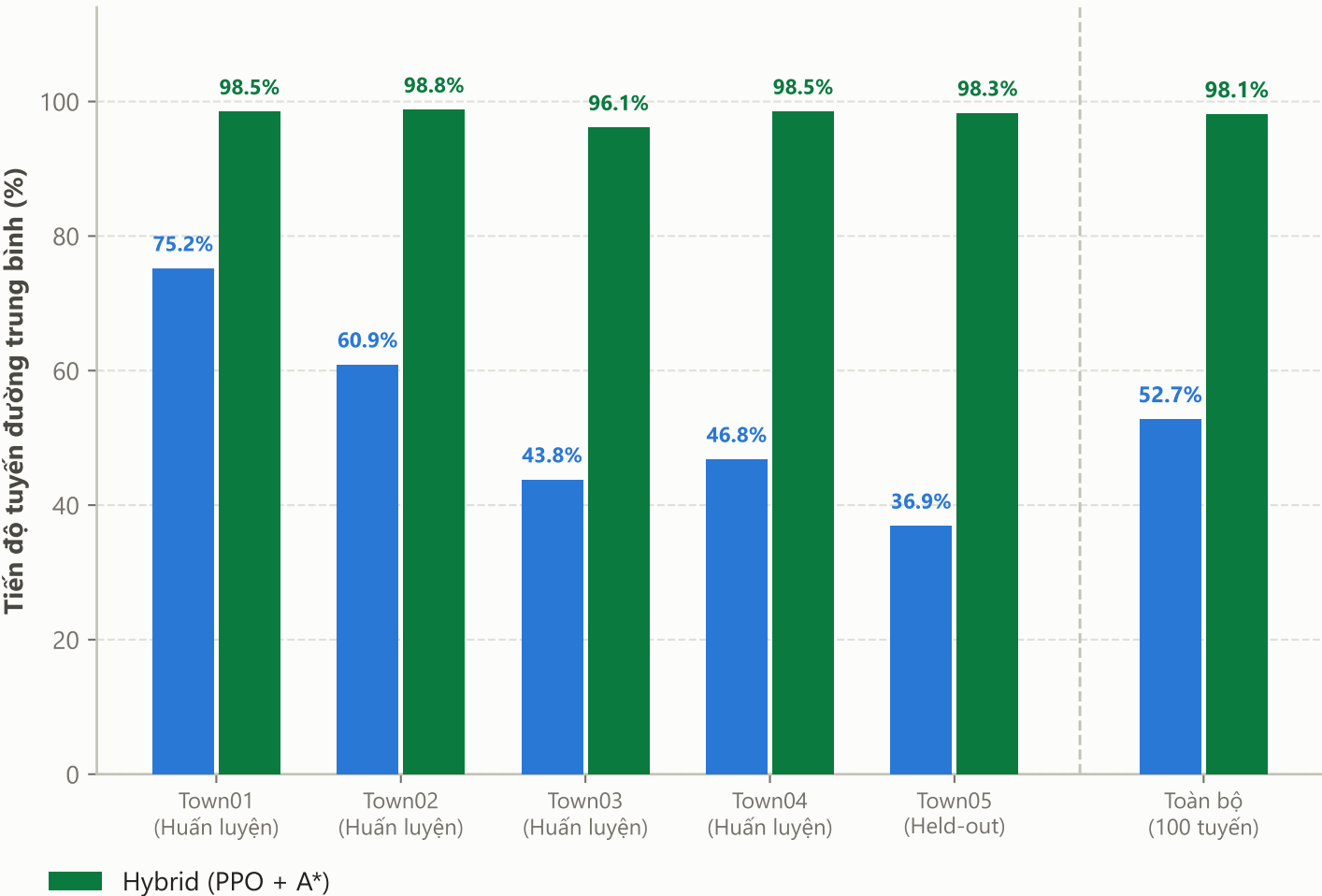
(b) Tiến độ hoàn thành chiều dài tuyến đường trung bình
