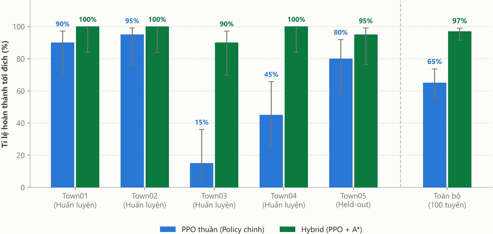
So sánh tỉ lệ hoàn thành tuyến đường (Tới đích thành công) PPO thuần vs. Hybrid (PPO + A*) trên các bản đồ CARLA (Thanh sai số: KTC Wilson 95%)
